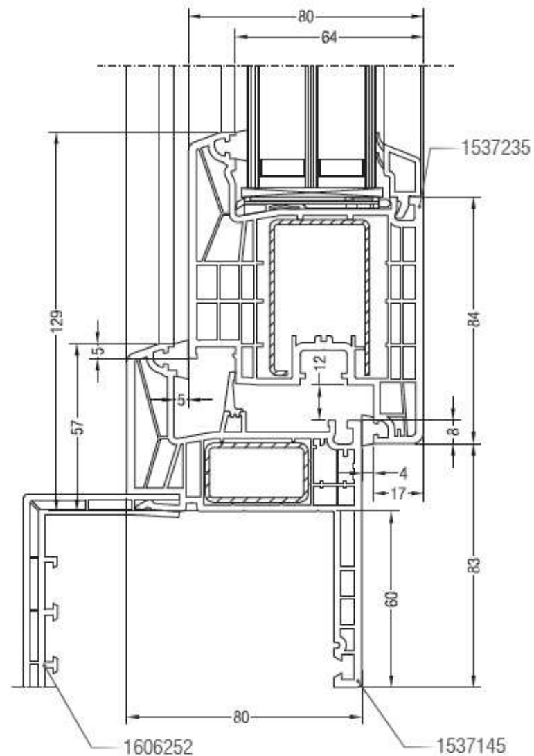
Sezione nodo anta dritta da 84 mm - telaio Z ( aletta da 60 mm )
