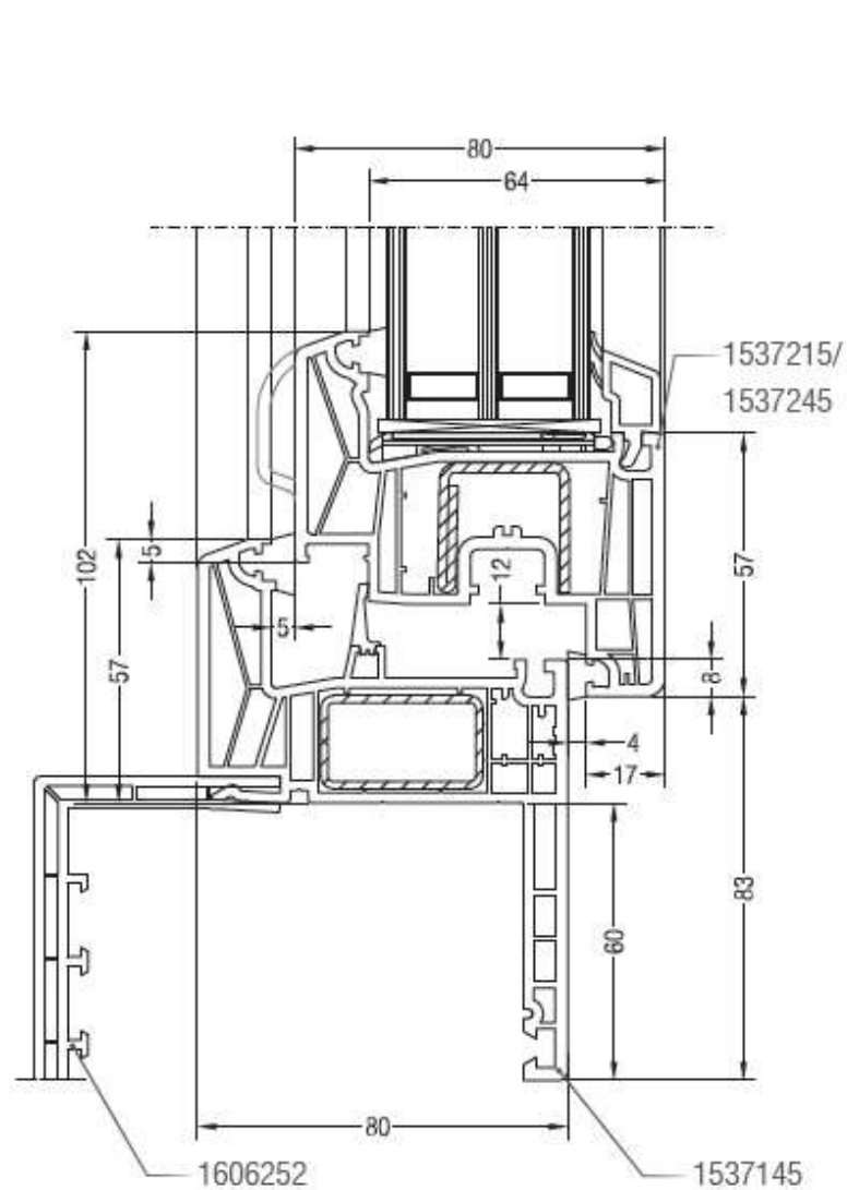
Sezione nodo anta arrotondata/dritta da 57 mm – telaio Z ( aletta da 60 mm )
